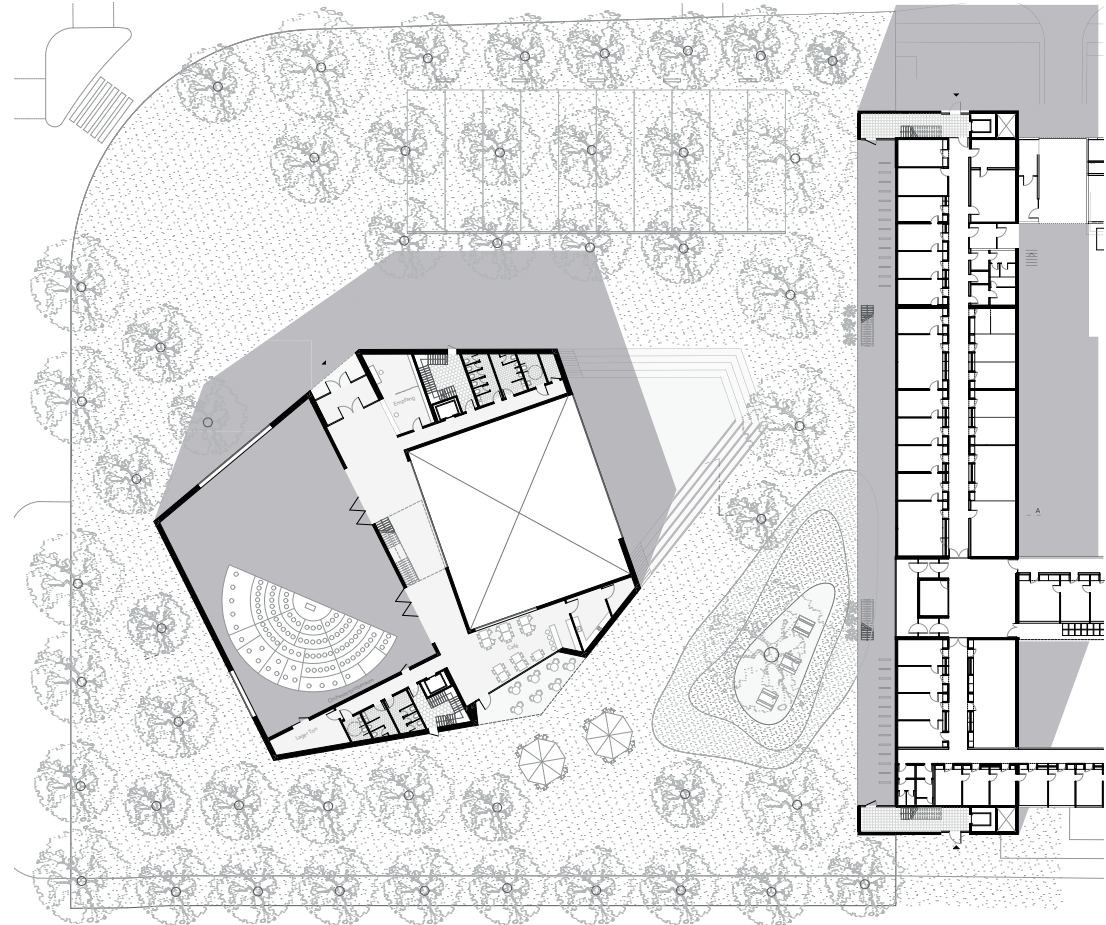
Grundriss | EG
