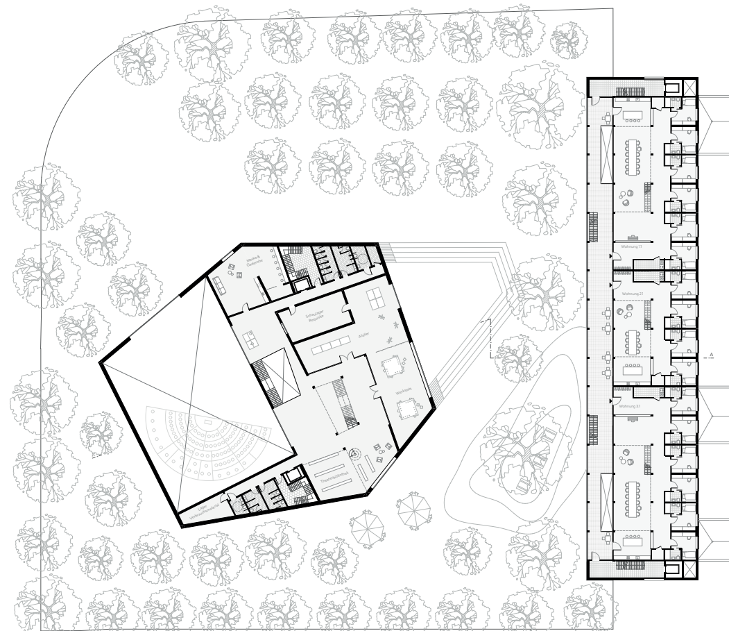
Grundriss | 1. OG
