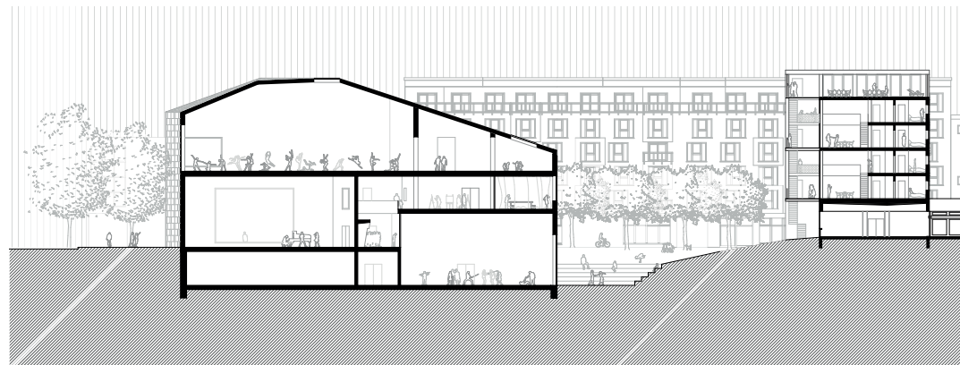
Schnitt
